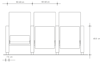
Vue de face — entraxe 50 ÷ 60 cm*
