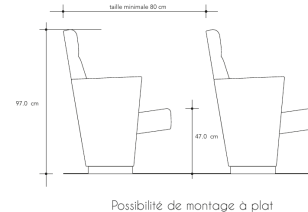
Montage à plat — encombrement minimal 80 cm*
